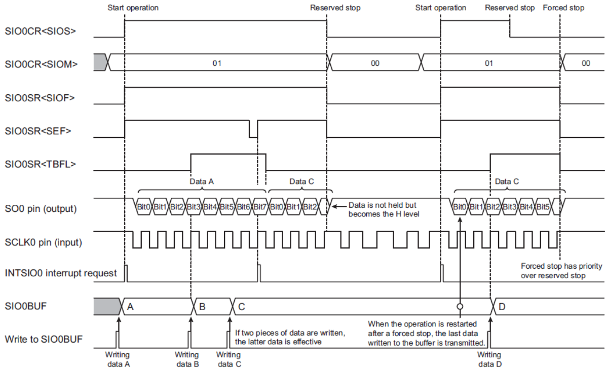
图 15-6 8 位元传送模式(外部时钟且强制停止)
