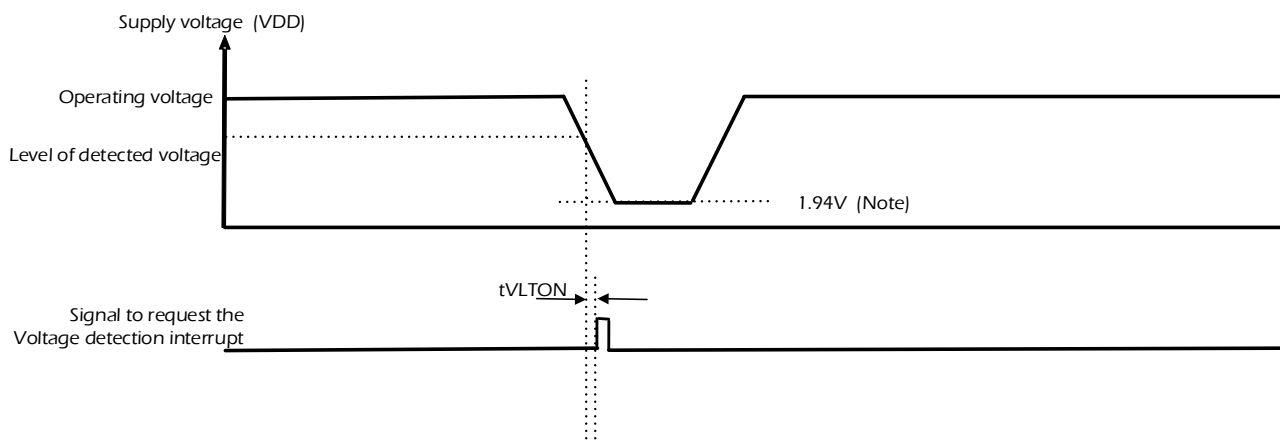
图 2-3 LVD 中断
