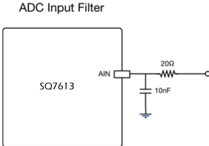
图 1-4 SQ7613 建议外部参考线路(进行 ADC 输入滤波)
