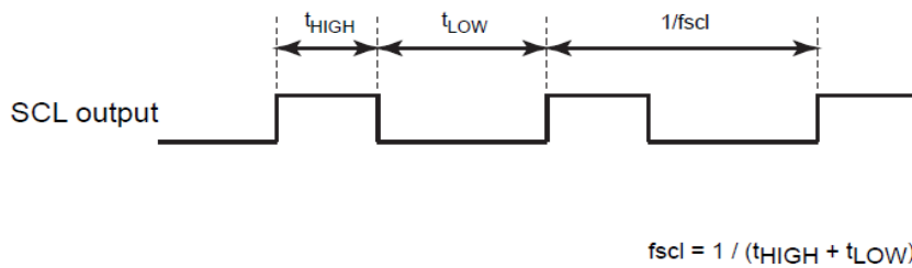
图 14-6 SCL 输出
