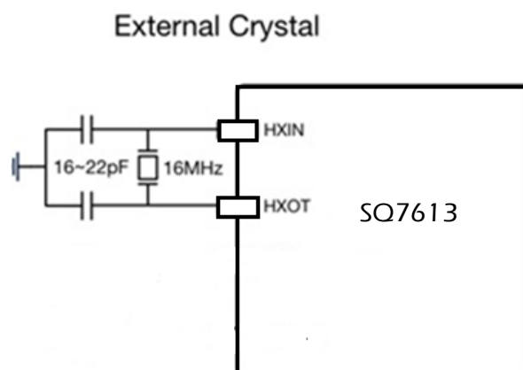
图 1-5 SQ7613 建议外部参考线路(使用外部参考时钟引脚)
