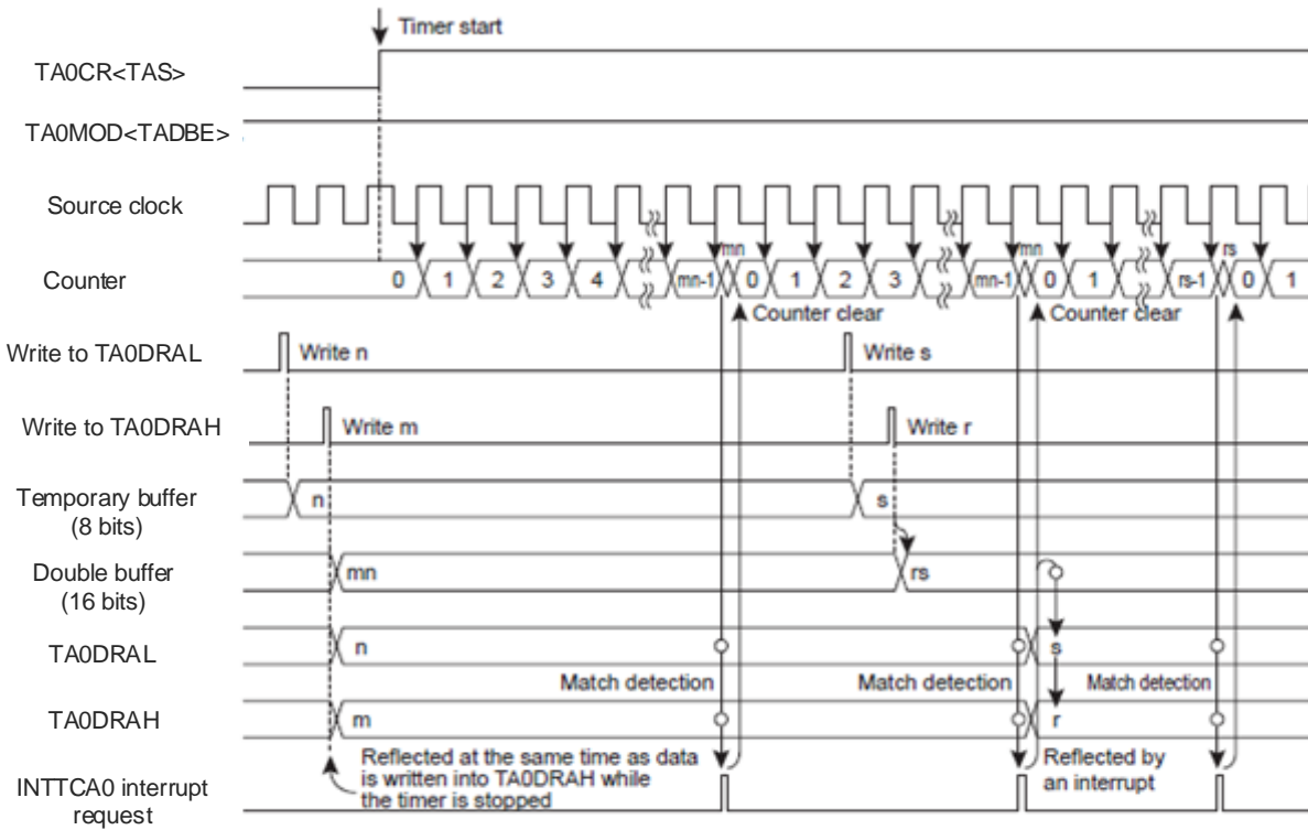
图 12- 10 定时器模式时序图(以 TCA0 为范例)
